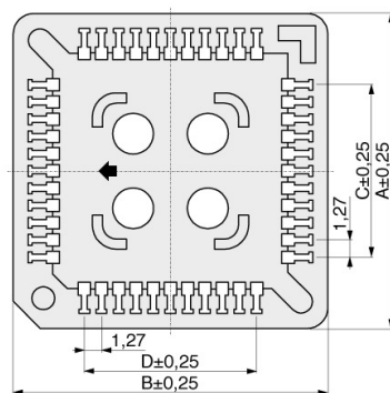
PIN 44 - 84
