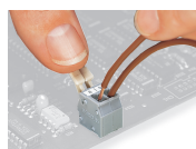
Leiter anschließen/lösen – mit Fingerdrückern, Betätigung von Hand – Serie 255.
