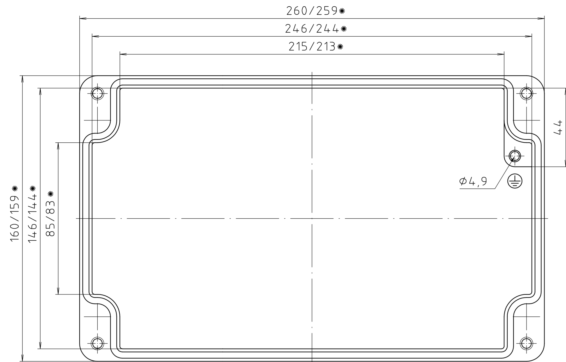
Deckel / lid
