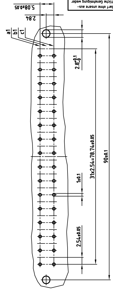
Leiterplattenbohrbild
