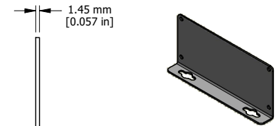
OPTIONAL FLANGE END PANEL 1455QF
