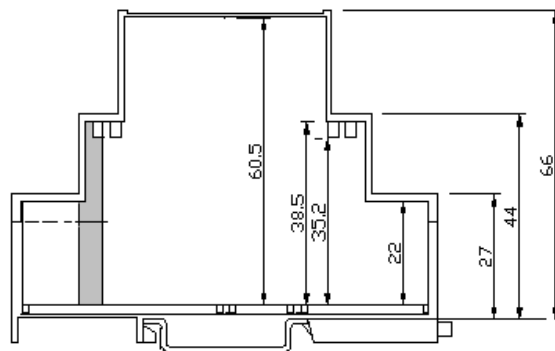
BARRA DIN
