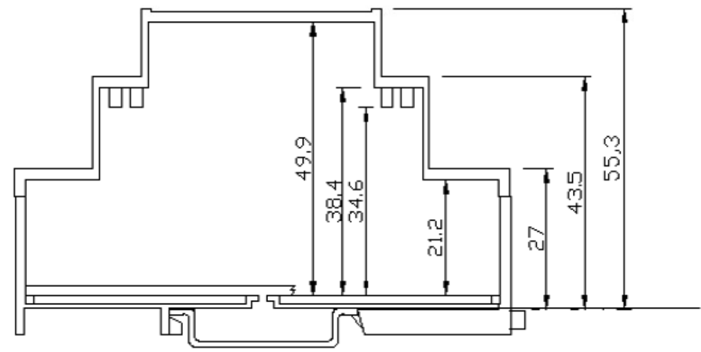
BARRA DIN
