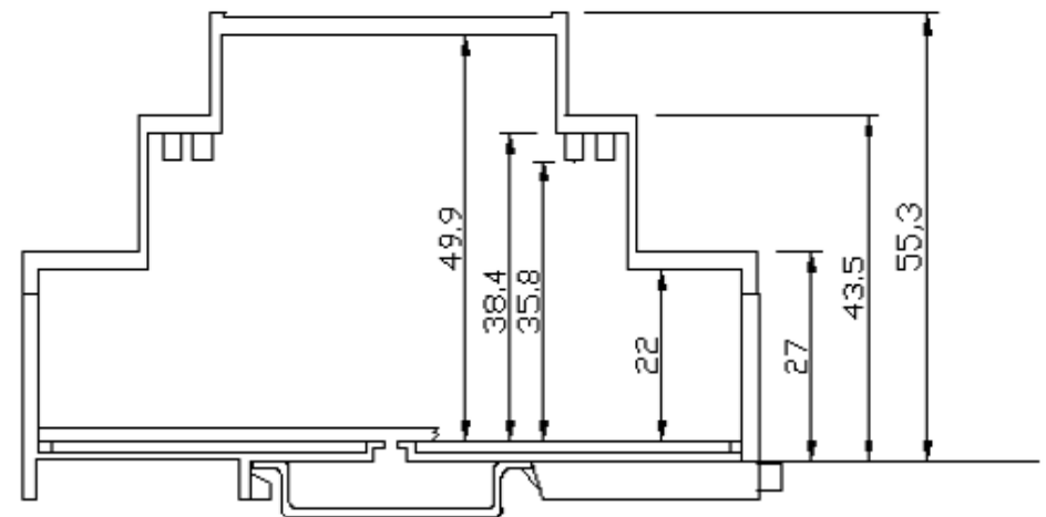
BARRA DIN
