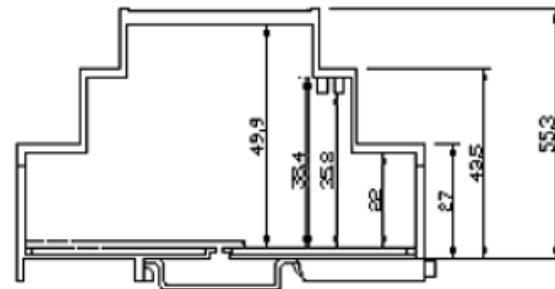
BARRA DIN
