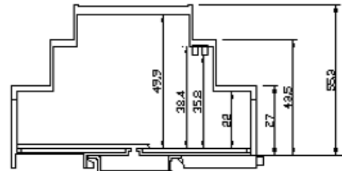
BARRA DIN
