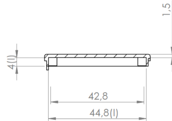
Sección/Section M-M
