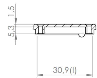
Sección/Section L-L
