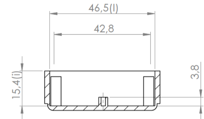
Sección/Section T-T
