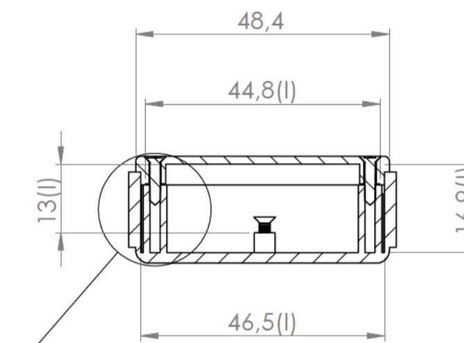
Sección/Section P-P
