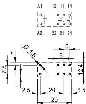
Ansicht auf die Anschlüsse
