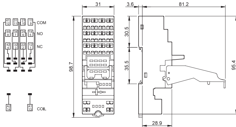
Fassung + Kammbrücke
