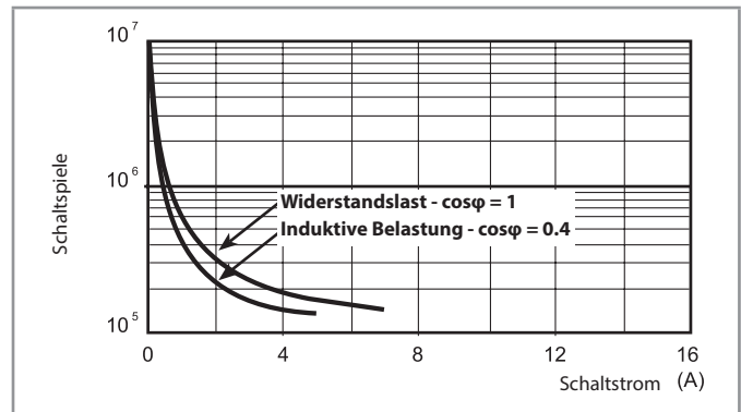
F 55 - Elektrische Lebensdauer bei AC 4 Wechsler
