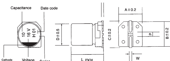
(φ 16:L±0.5)
