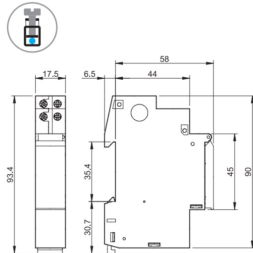
Typ 12.11 Käfigklemmen
