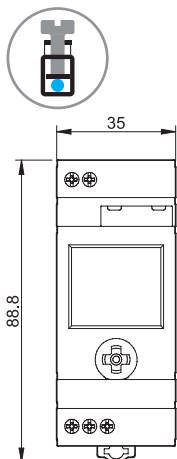
Typ 12.51/12.81 Käfigklemmen
