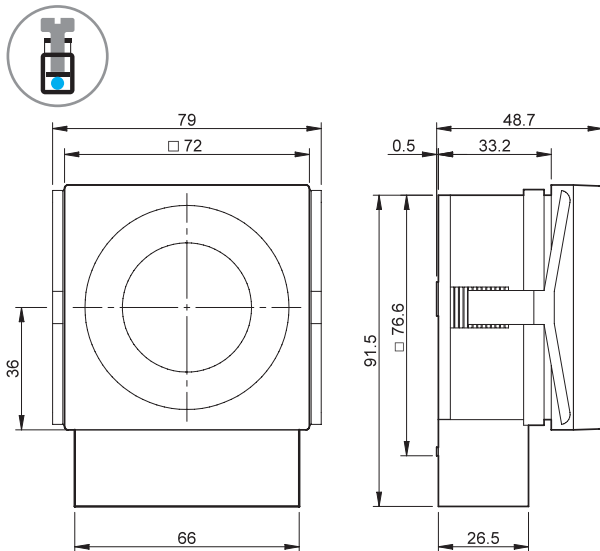
Typ 12.31 Käfigklemmen
