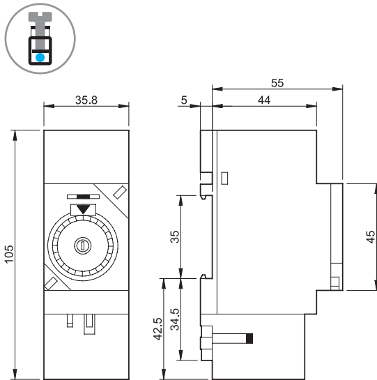
Typ 12.01 Käfigklemmen
