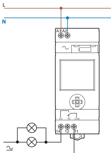
Typ 12.51 und 12.81
