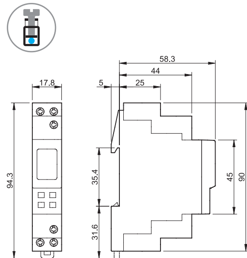
Typ 12.71 Käfigklemmen
