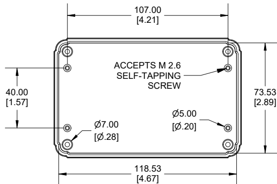
INSIDE LID
