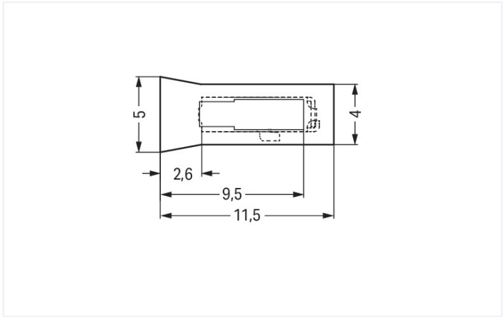
Abmessungen in mm Benötigter Raum für Betätigungswerkzeug
