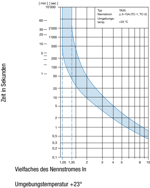
Auslösekennlinien thermisch I_n \geq 3 \dots \leq 15\text{ A}
