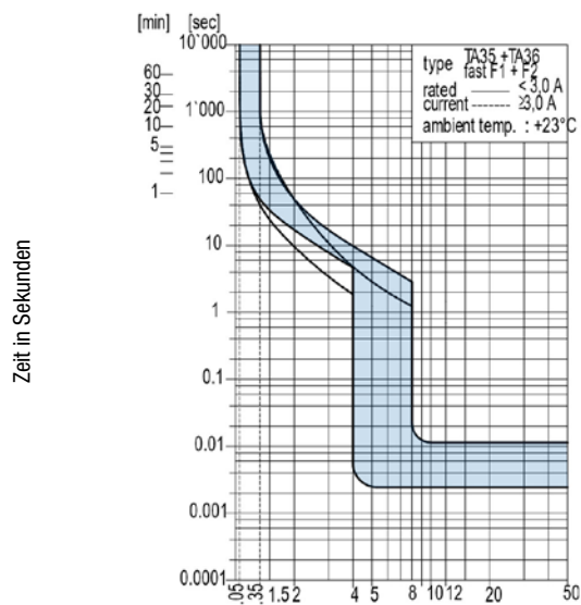
Auslösekennlinien thermisch magnetisch flink
