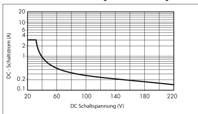
H 7S16/36 - Gleichstromschaltvermögen bei DC13-Belastung - 7S.16/36
