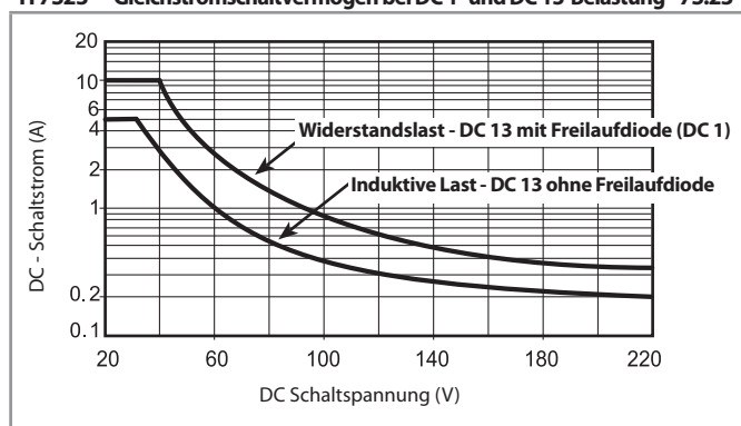
H 7S23* - Gleichstromschaltvermögen bei DC 1- und DC 13-Belastung - 7S.23
