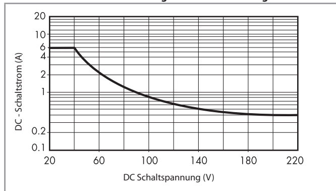
H7S16* - Gleichstromschaltvermögen bei DC 1-Belastung - 7S.16/36
