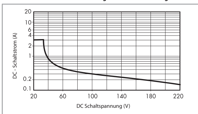
H 7S14/34 - Gleichstromschaltvermögen bei DC13-Belastung - 7S.14/34
