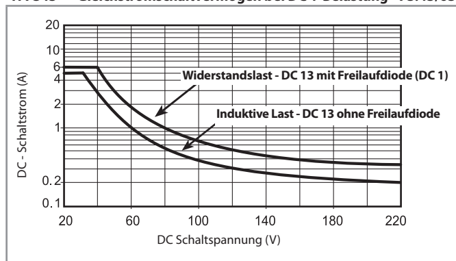
H 7S43* - Gleichstromschaltvermögen bei DC 1-Belastung - 7S.43/63
