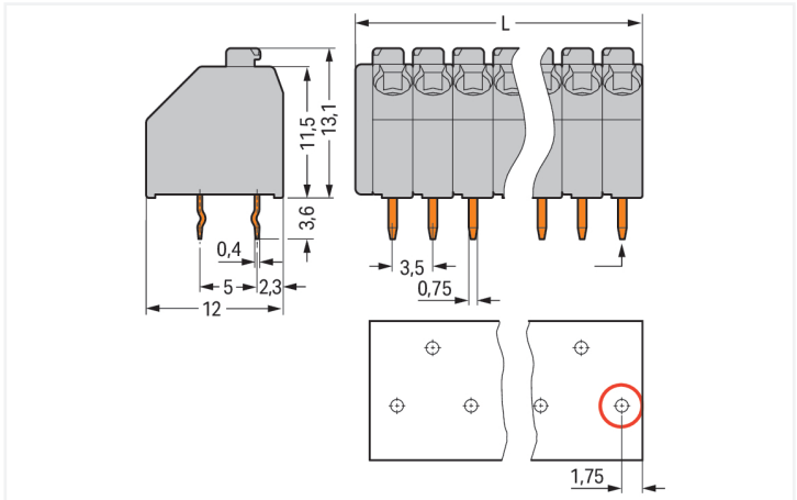
Abmessungen in mm L = (\text{Polzahl} \times \text{Rastermaß}) + 1,5 \text{ mm} (roter Kreis) erster Lötstift vorne rechts
