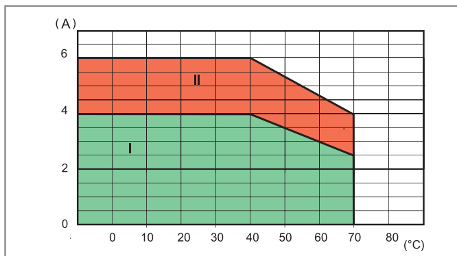
L 39 - Dauerstrom-Belastbarkeit - Dauerstrom in Abhängigkeit von der Temperatur
