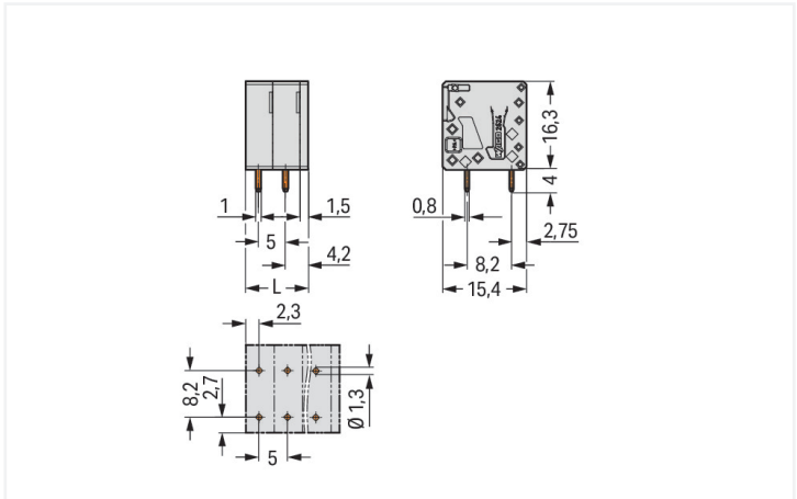
Abmessungen in mm L = (\text{Polzahl} - 1) \times \text{Rastermaß} + 6,5 \text{ mm}
