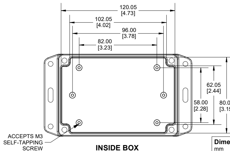
BOTTOM BOX
