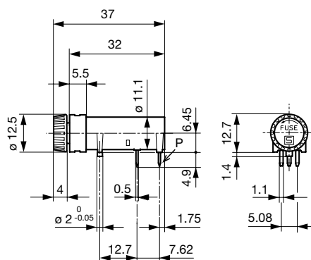
Variante Fingergrip 3101.0055 / Steckanschluss verzinkt
